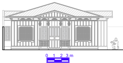
Elevation 01
